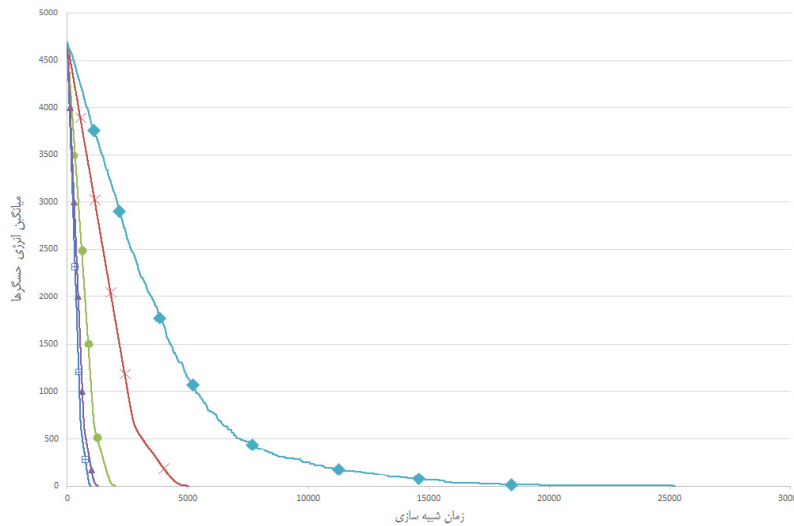
شکل ۹: مقایسه میانگین انرژی حسگرها در الگوریتم‌های مختلف.
